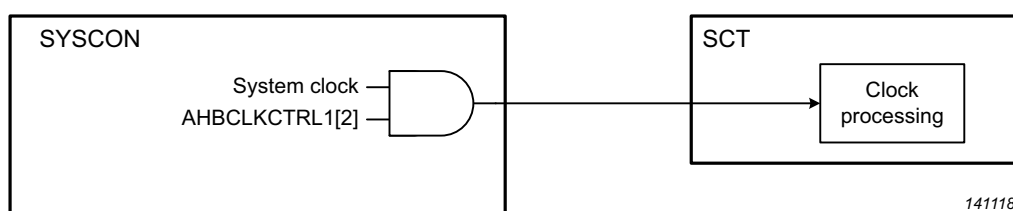
Fig 20. SCT clocking
